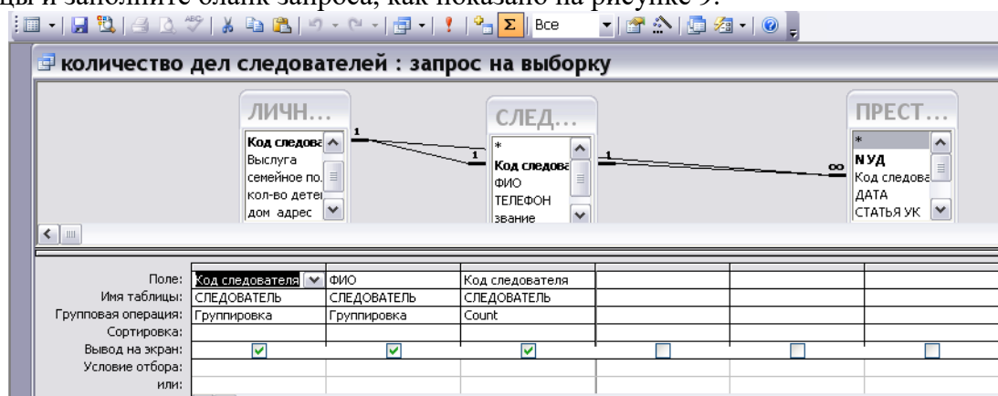
Рис.9 Бланк запроса
